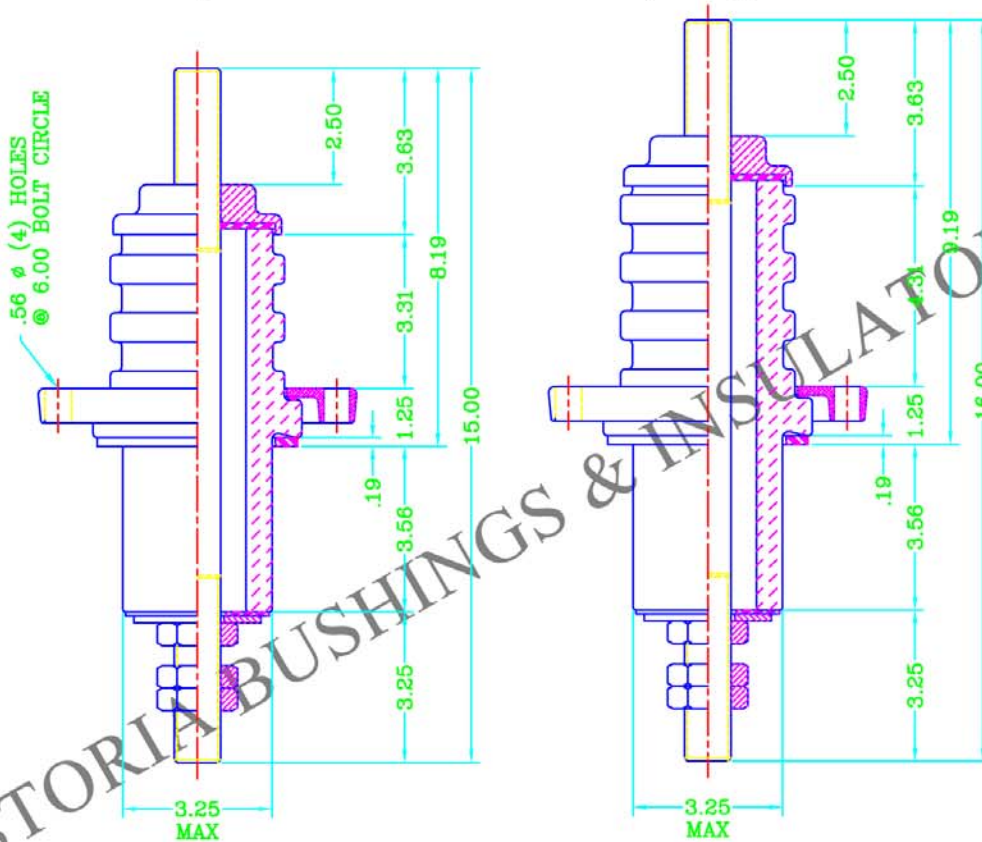
2.5 kV CLASS LEAKAGE DISTANCE 4.00" MIN.
